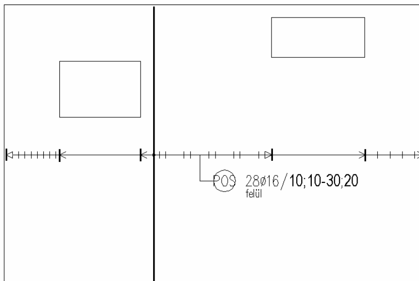
Allértra bontás szakasz osztásközök segítségével
