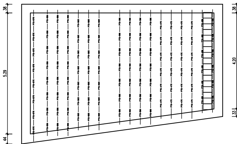
Egyetlen sor béléstest behelyezése a szélső gerenda mellé
