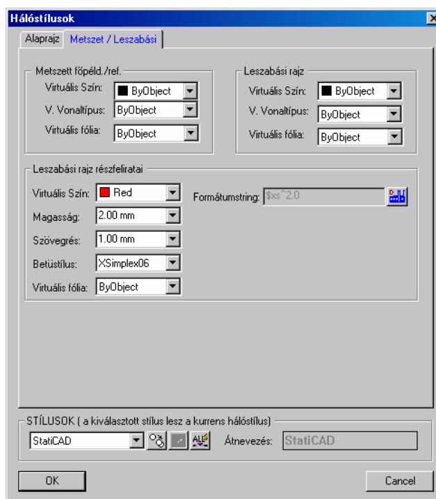
A Leszabási rajz típusú referenciák megjelenését befolyásoló paraméterek
