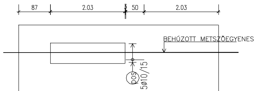
Kótasor, ha egy KiosztásiVonalat metszünk el
