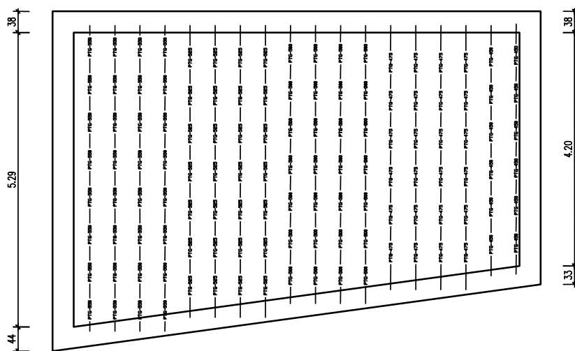
A Nyújtás után öt különböző hosszúságú (PTG-450-től PTG-570-ig terjedő) gerendacsoport keletkezett
