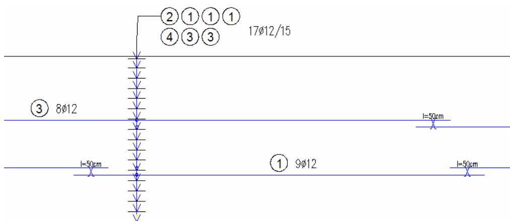
Átfedési hézag és Átfedési blokk a toldásoknál
