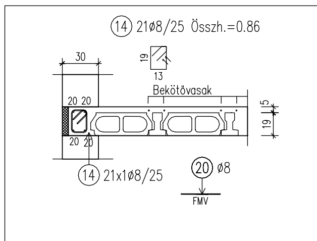
Részlet objektum, melyre a rajzban több helyen hivatkozhatunk
