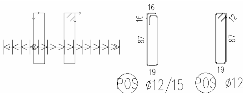
8 mm átmérőjű kengyel kampói 90 és 135 fokos hajlásszög esetén a leszabási rajzon
