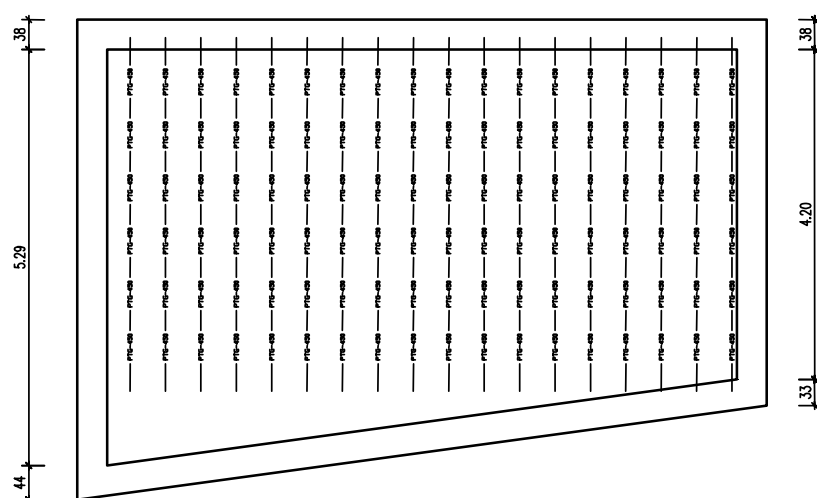
PTG-450-es jobbról egyenletesen kiosztva Nyújtás előtt
