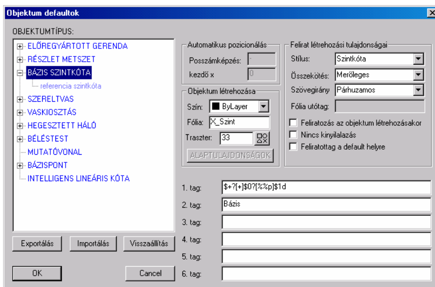
Bázis-szintkóta alapértékei az Objektum defaultok között
