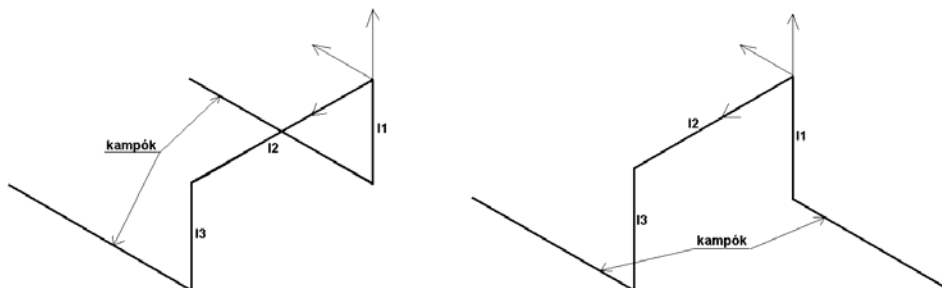
Két előregyártott térbeli kampós vas – rövid konzol és számlivas - axonometrikus nézetben
