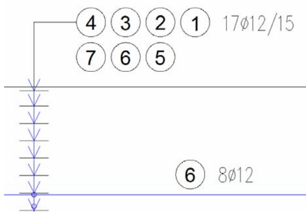
POSmátrix a létravégén a Multivasnál
