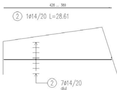
VÁLTOZÓ HOSSZÚSÁGÚ VASAK
