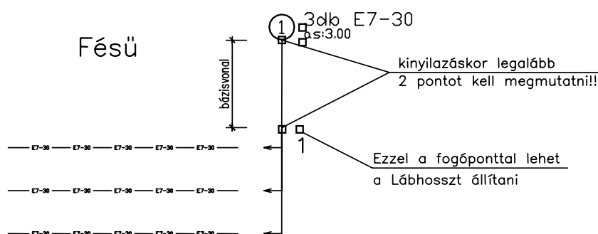
Fésű kinyilazás –5,0-ös alap Lábhosszal
