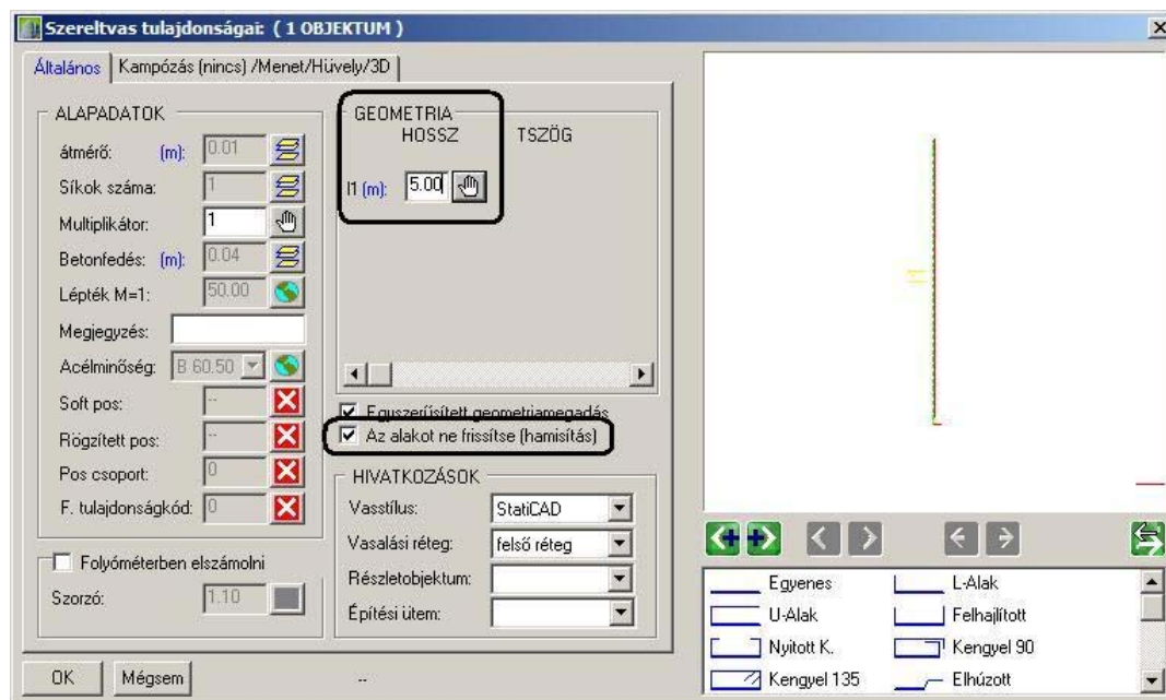
Vas hamisítás a tulajdonságpanelen történik
