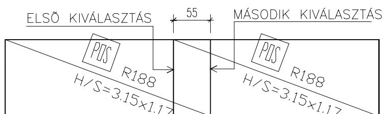
Hegesztett Hálók toldásának kótázása
